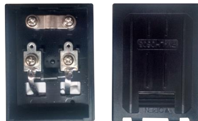
Terminales de conexión
